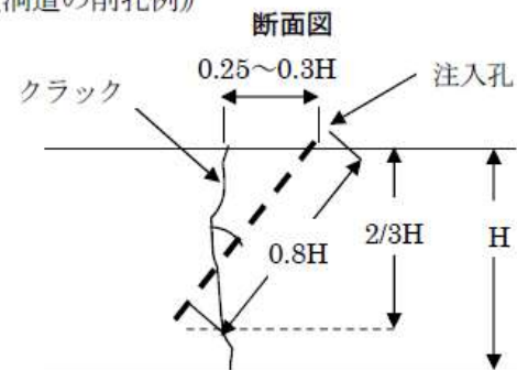
《洞道の削孔例》
