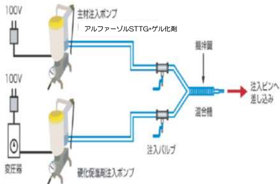
図ー1 STTG工法機器構成の概要
