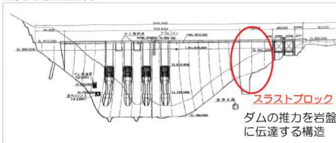
正面図（上流より望む）
