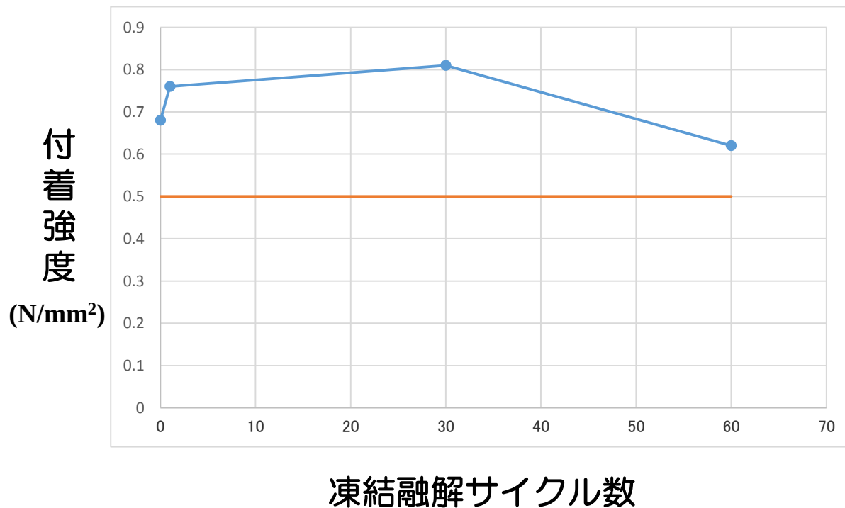
図ー3 凍結サイクル数と付着強度との関係
