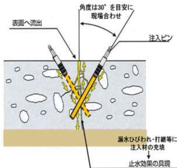
図-3 止水材充填のイメージ
