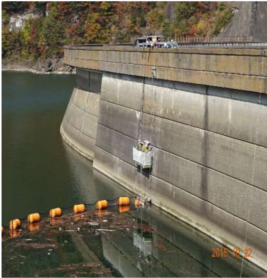
施工中（全景）
