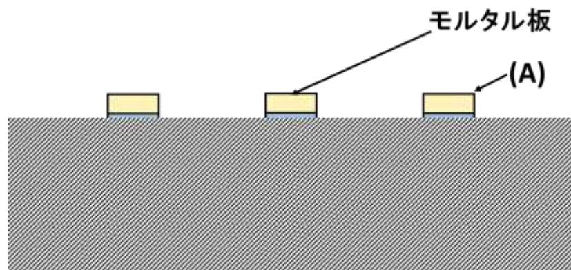
図ー2 モルタル板への吊上げ金具の取付け
