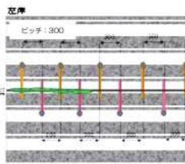
ダム上流面
